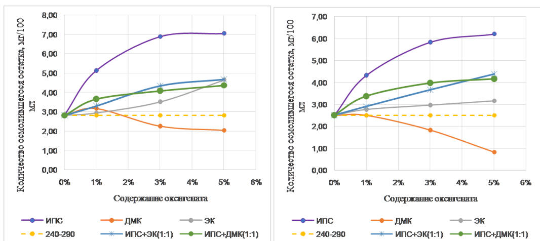
Рис. 2. Зависимость количества осмолившегося остатка при 225°C и 280°C от типа и содержания кислорода во фракции 240-290°C
