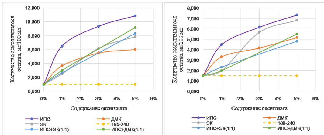
Рис. 1. Зависимость количества осмолившегося остатка при 225°C и 280°C от типа и содержания кислорода во фракции 180-240
